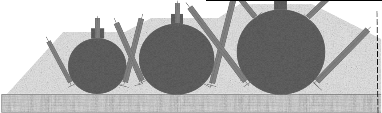
Figura B1e – Esempio di possibili configurazioni adottabili per serbatoi con profilo di attenuazione fortemente condizionante o con diametro maggiore di 4,5 metri.
