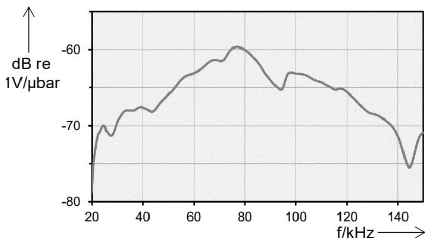
Figura 3 - Curva di risposta in frequenza di un sensore EA con frequenza di picco 75 kHz
